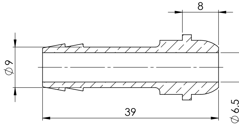
Ansicht / view A-A
